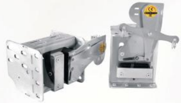
Fren Bloğu ( Safety Gear )
